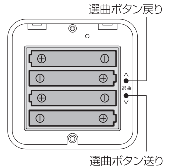
押しボタン送信機
