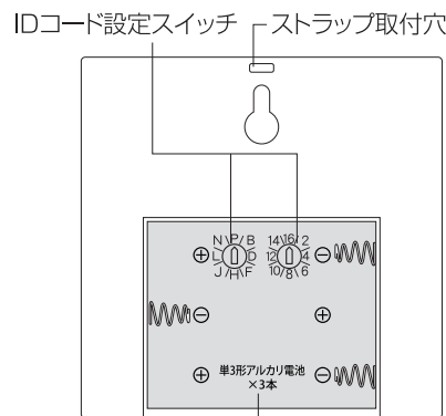
電池BOX
